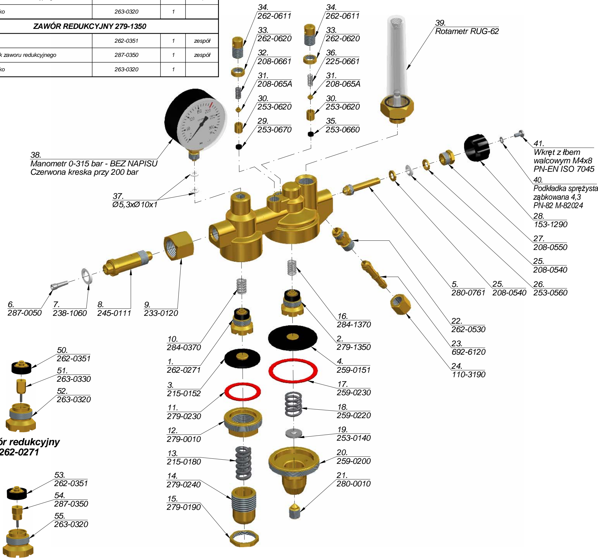
Zawór redukcyjny 279-1350
