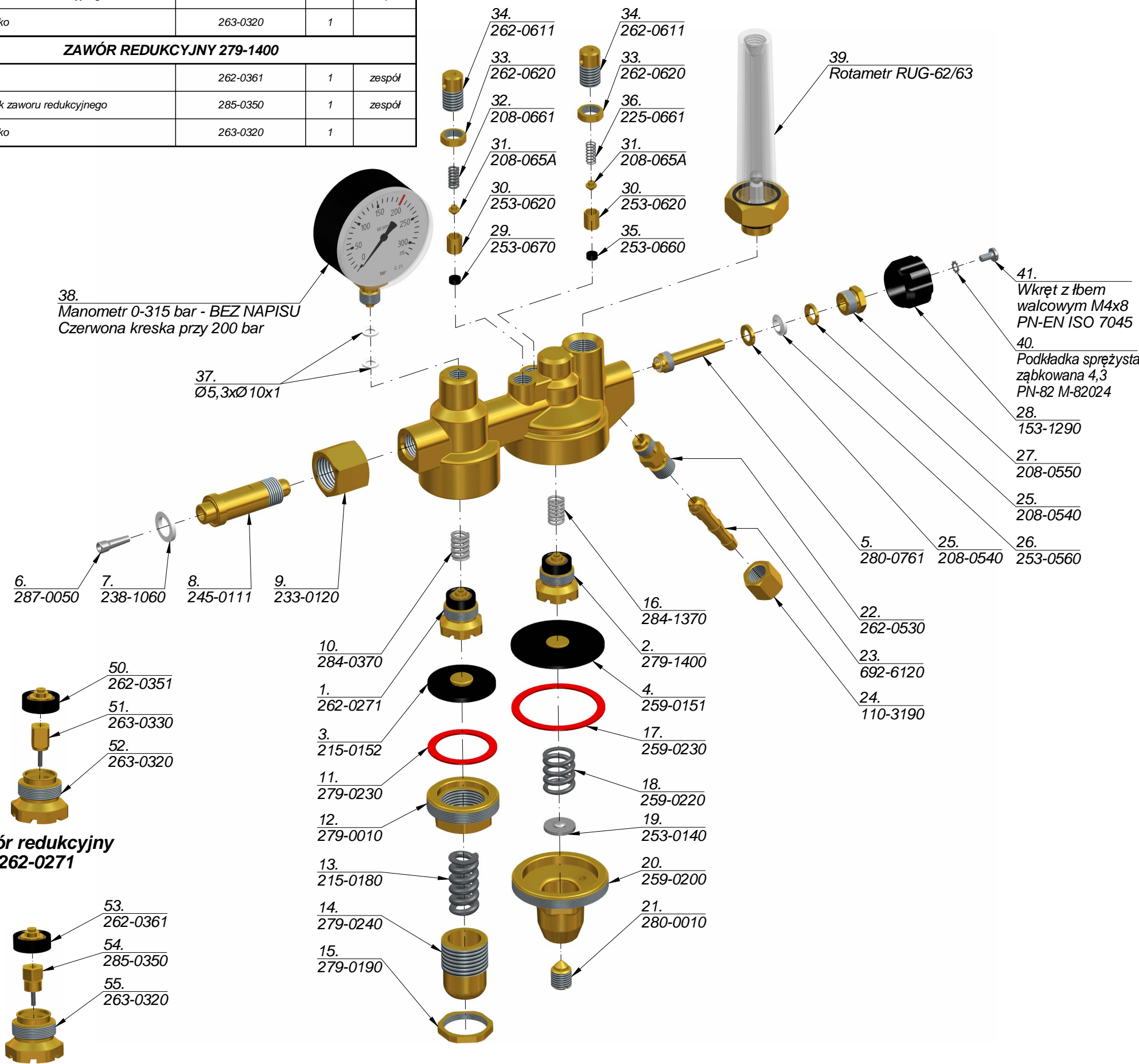
Zawór redukcyjny 279-1400
