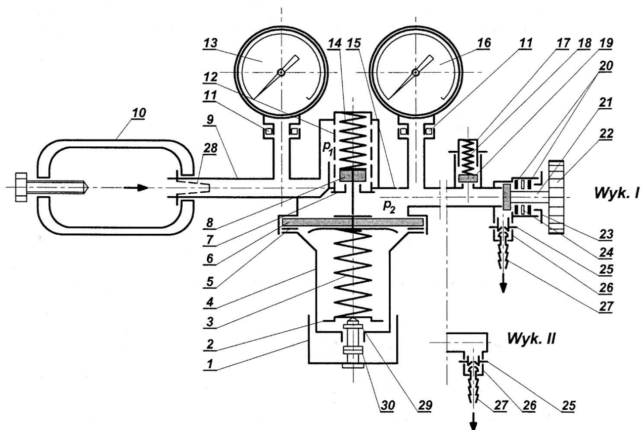
SCHEMAT REDUKTORÓW JEDNOSTOPNIOWYCH DO ACETYLENU:
